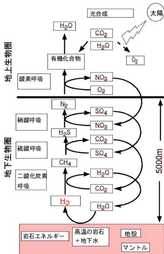
補足図 1. 地下生物圏における水素の産生。地下の玄武岩のような岩が、帯水層の水を還元して水素分子を作り出す。地下 5,000 メートルまで生息している多くの岩石栄養生物は水素分子を化学呼吸系によってメタン、硫化水素と窒素へ酸化する。ある種の地下水は多くのミネラルナノ粒子とミネラルナノ粒子水素化物を含んでいる可能性がある。はニュートン誌の論文の図を一部修正した (Newton editorial 2001)。
